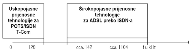
Slika 1. Frekventijski obim za uskopojasne i širokopolasne prenosne tehnologije
